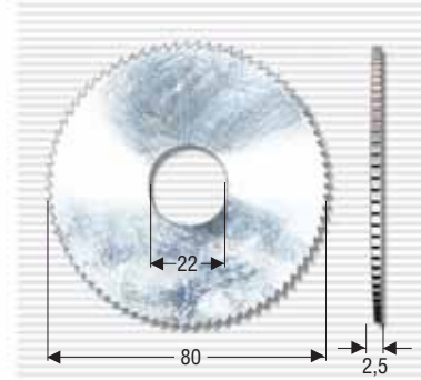
ABUS 07614 07605 Fräser 2 + Taster 2 Cutter 2 + Tracer 2 Fraise 2 + Palpeur 2 SKM 5000-2 für/for/pour Bahnen-Schlüssel Laser type keys Clé à vague
