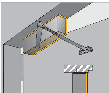
Sturzfutterwinkel
