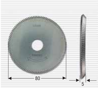
ABUS 03680 Fräser · Cutter · Fraise SKM 2500-1 + SKM 3000-1
